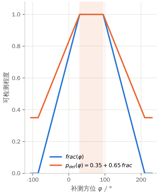
(b) 衰减是线性的，且有 0.35 的先验托底
