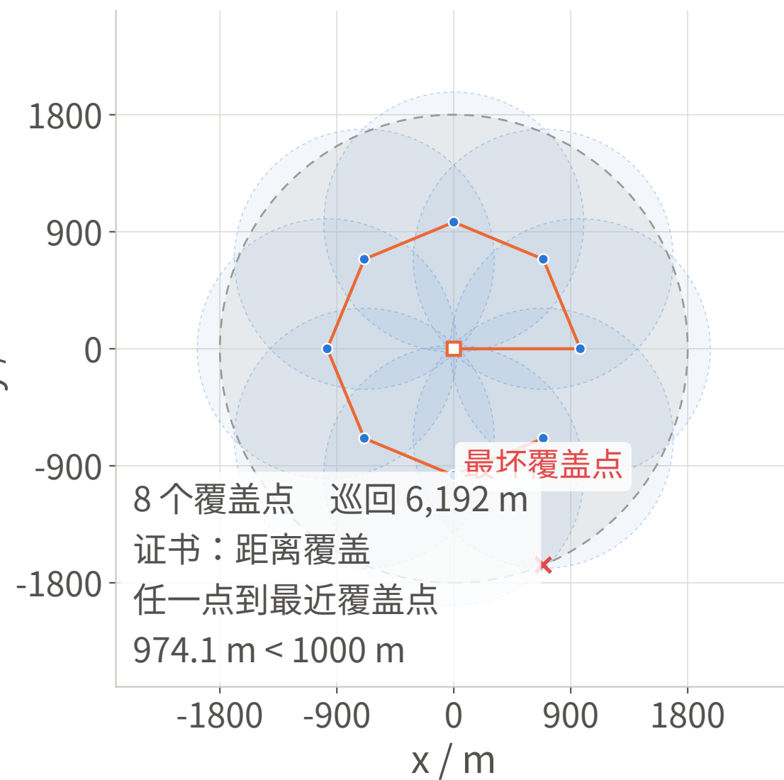
(a) 问题三 正八边形覆盖网
