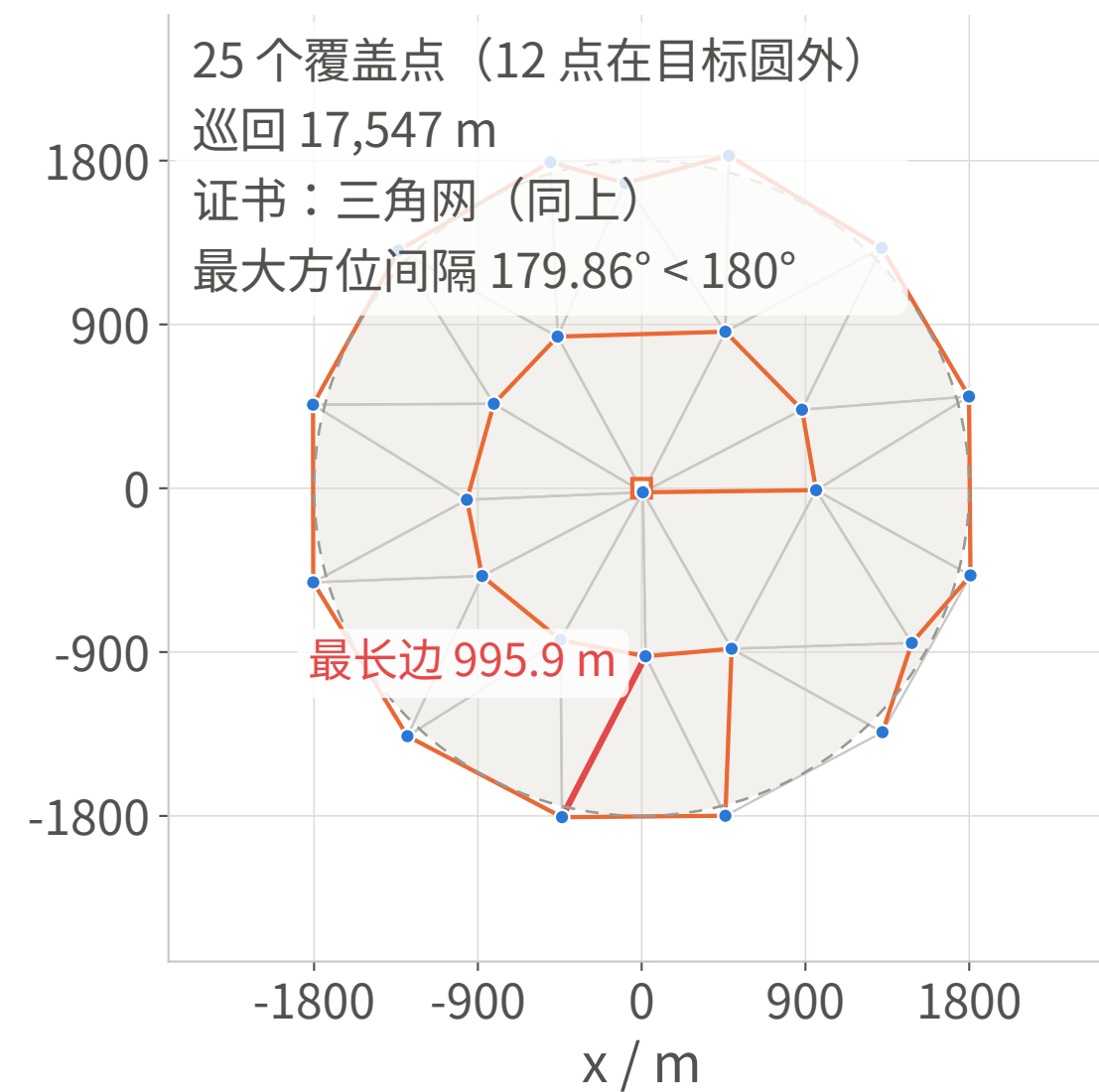
(c) 问题四·方案七 非规则三角网
