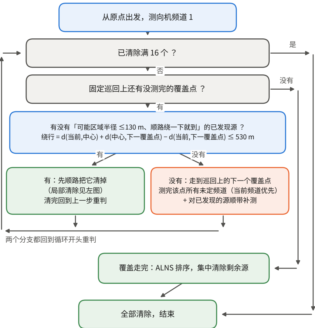
(b) 主循环 (方案四：固定巡回 + 顺路清除 + ALNS 收尾)
