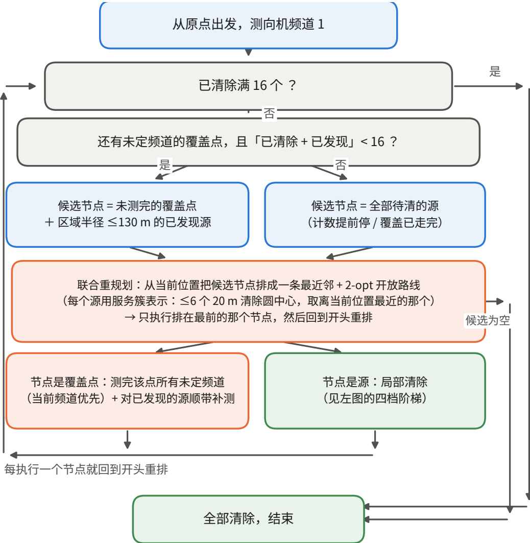
(b) 主循环 (方案七：联合重规划 + 服务簇 + 计数提前停)
