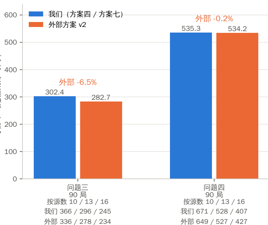
(c) 常规随机案例：问题三他们更快，问题四打平
