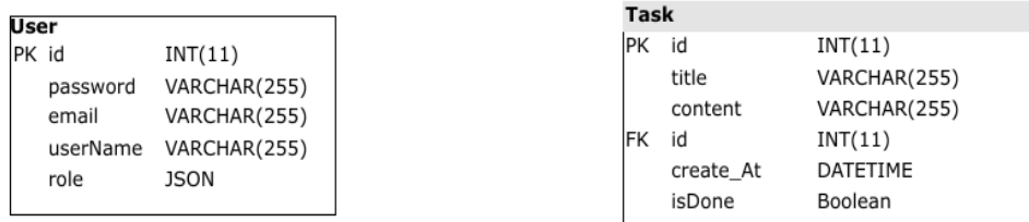
Figure 1 : Diagrammes de classe
