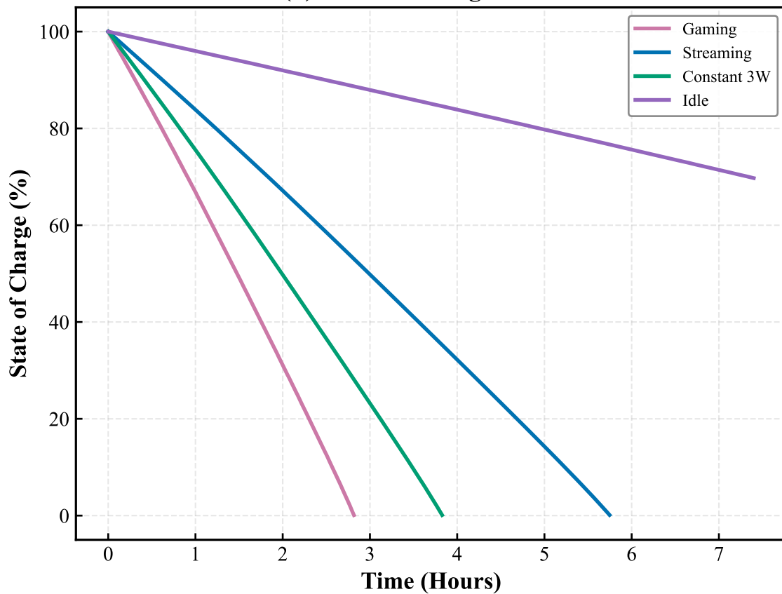
(d) TTE Comparison
