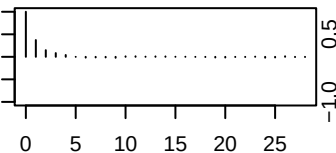
mu
