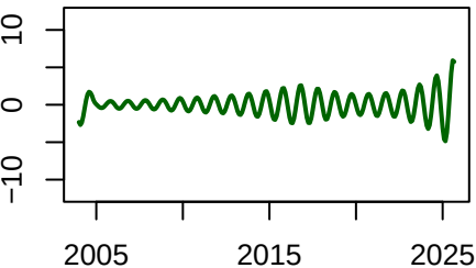
period=12
