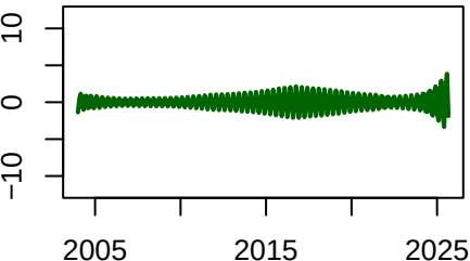
period=4
