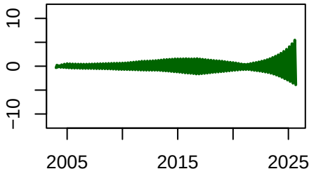
period=3
