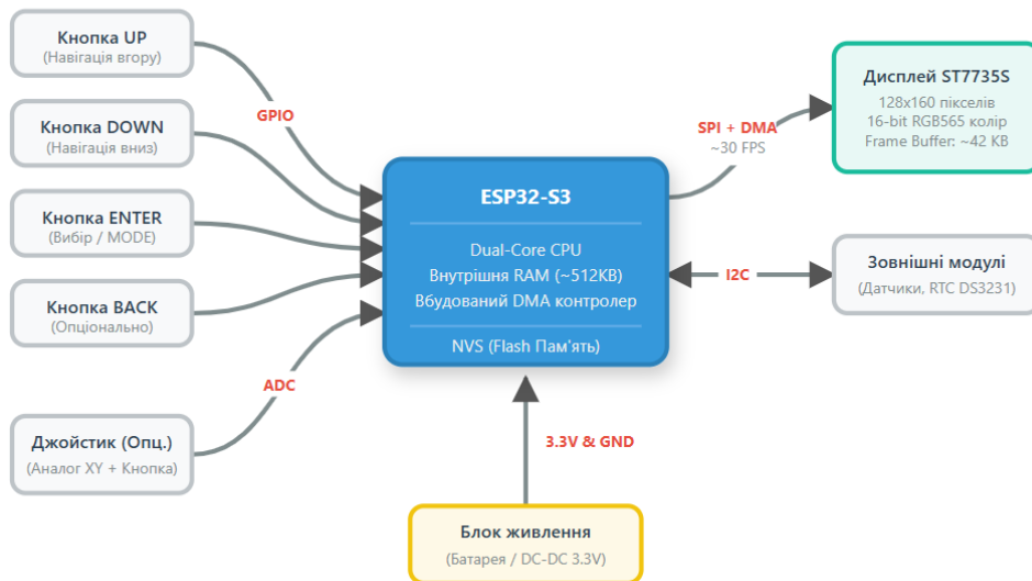
Блок-схема апаратної архітектури ESP32-S3 (Дисплей ST7735S)
