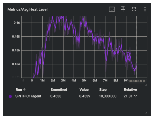
Σχήμα 25: Μέση θερμοκρασία πράκτορα (Πείραμα 3)
