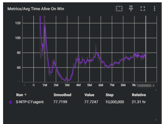
Σχήμα 29: Διάρκεια επεισοδίου σε νίκη πράκτορα (Πείραμα 3)
