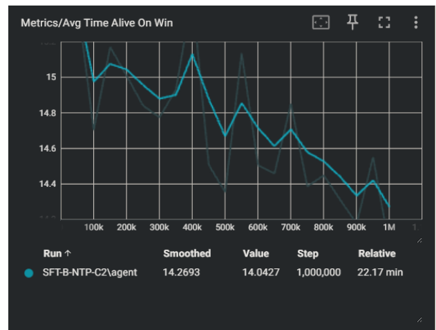
Σχήμα 38: Διάρκεια επεισοδίου σε νίκη πράκτορα (Πείραμα 4)
