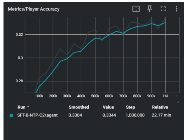
Σχήμα 36: Ακρίβεια βολών πράκτορα (Πείραμα 4)
