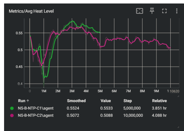
Σχήμα 7: Μέση θερμοκρασία πράκτορα (Πείραμα 1)
