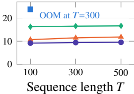
Peak VRAM (GB)
