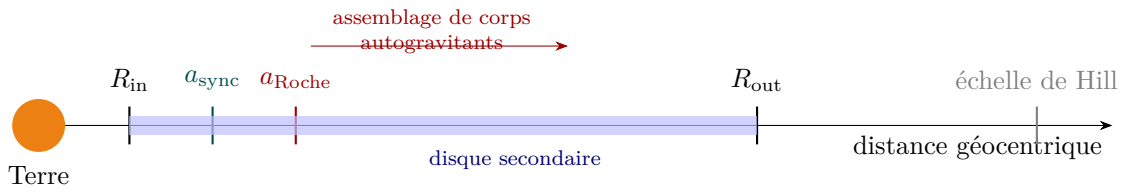
FIGURE 10.1 – Organisation radiale conceptuelle du disque circumterrestre. Les rayons interne, synchrone, de Roche, externe et de Hill jouent des rôles physiques différents (échelle non respectée).
