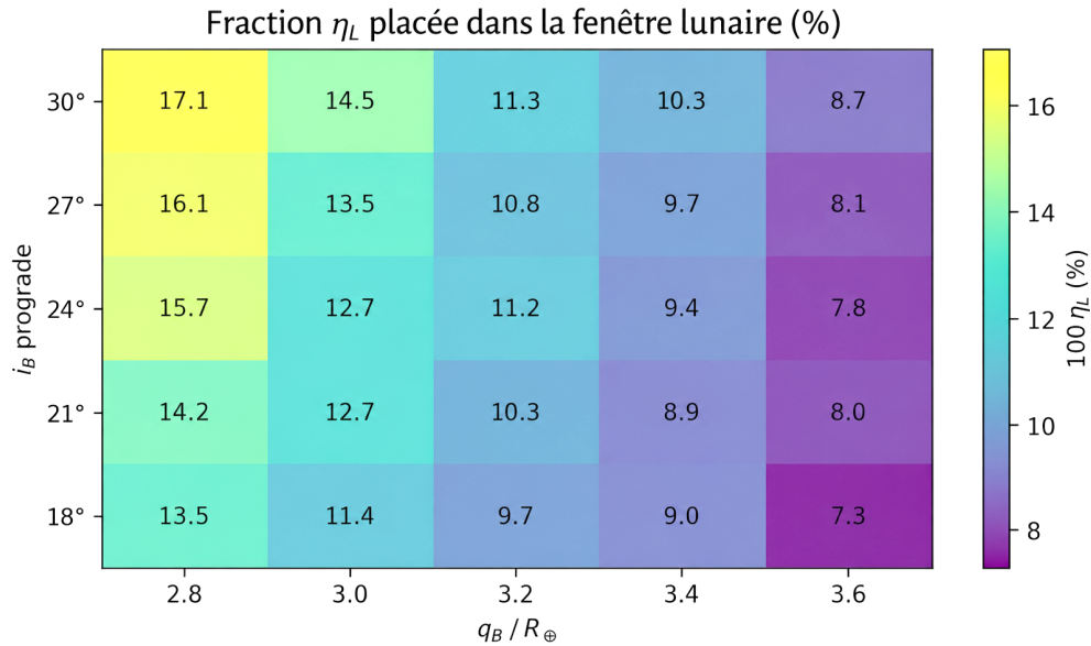
FIGURE 16.2 – Carte pilote de \eta_L(q_B, i_B) pour le cas M_B = 0,10 M_{\oplus} , v_{\infty} = 2 \text{ km s}^{-1} et \omega_B = 90^\circ . La carte illustre l'existence d'une bande de réponses continues, à confirmer par des simulations massives, collisionnelles et autogravitantes.
