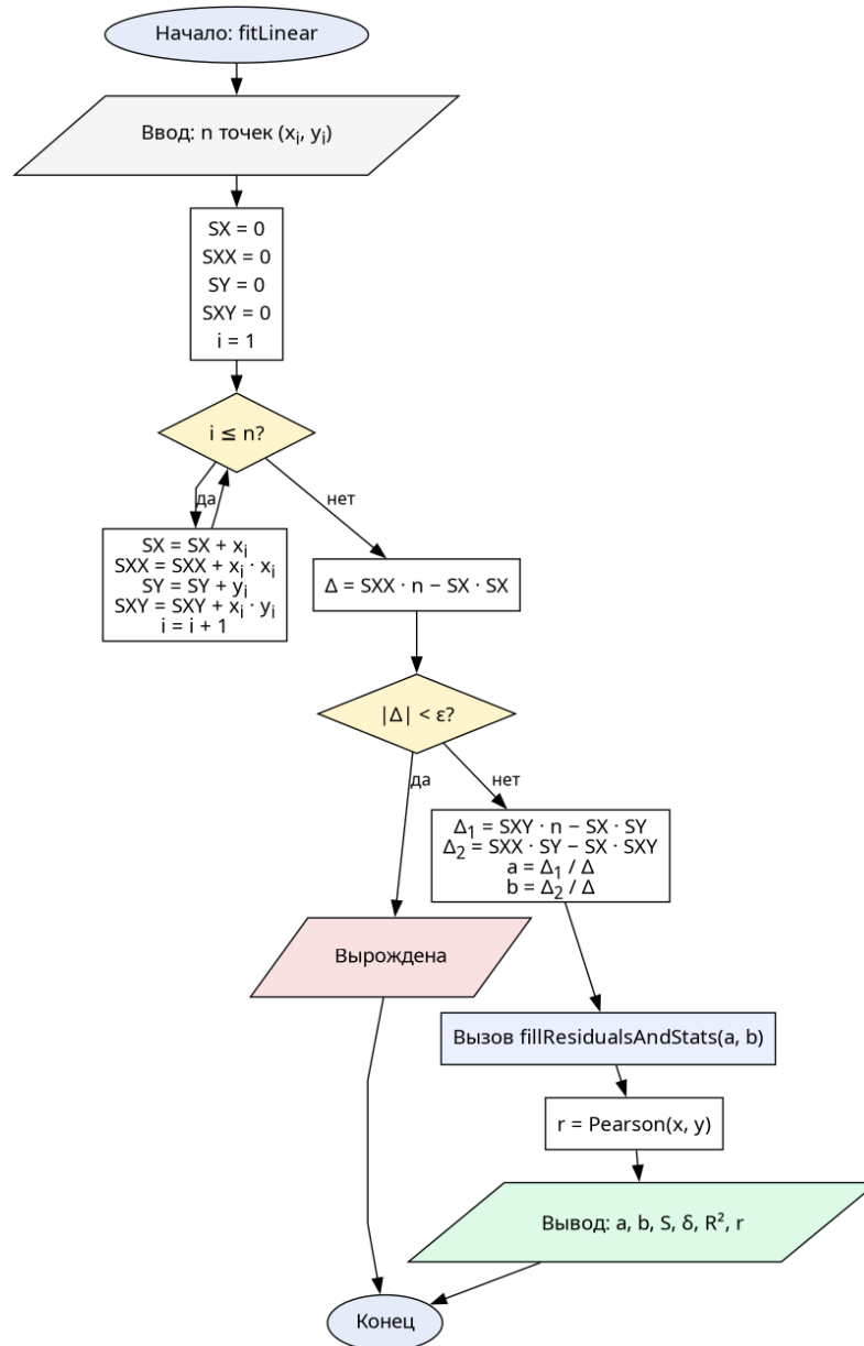
Рис. 1. Блок-схема линейной модели
