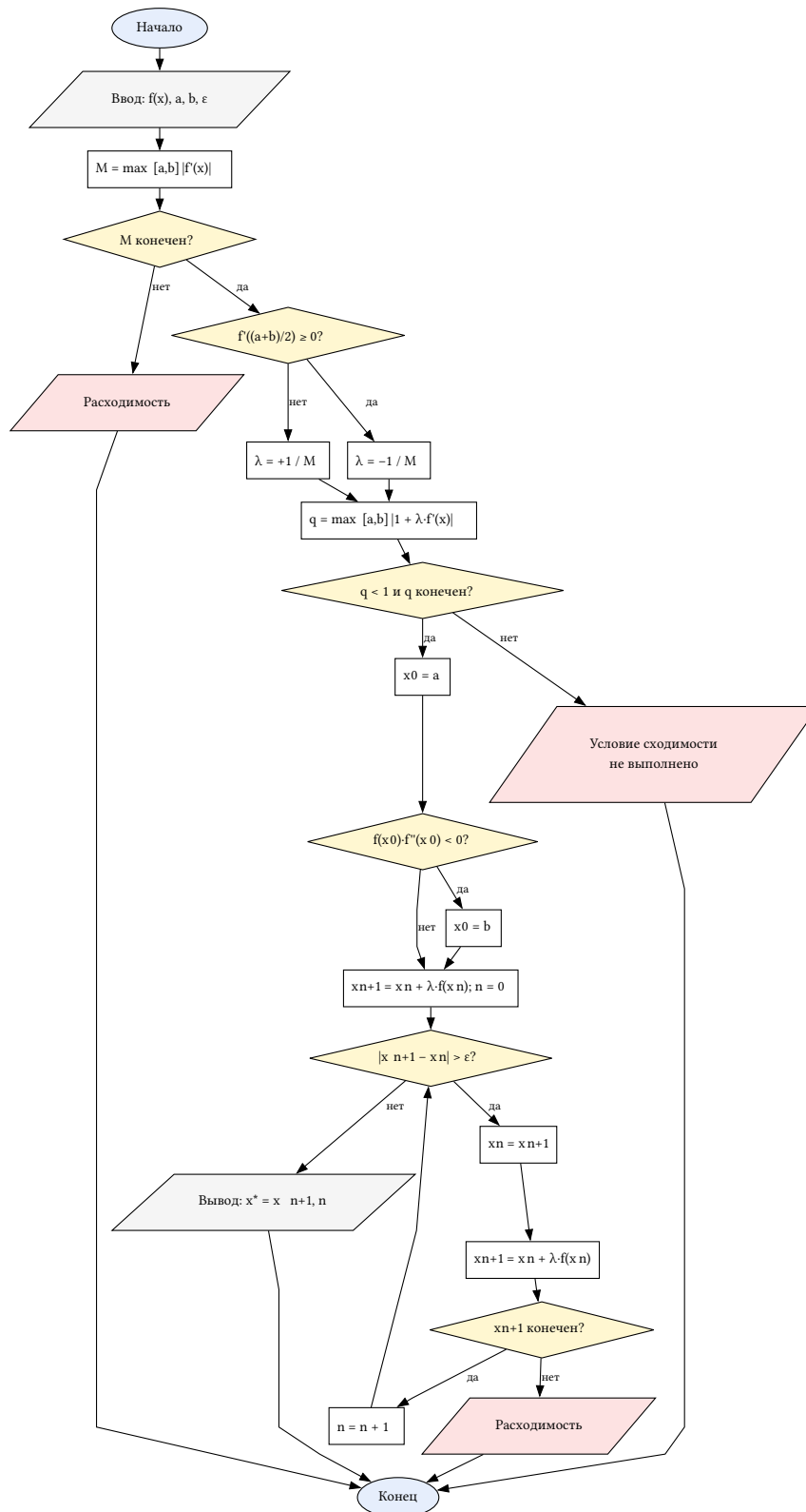
Рис. 3. Блок-схема метода простой итерации для уравнения 2.1.4 Метод простой итерации (для системы) Исходная система приводится к эквивалентному виду:
