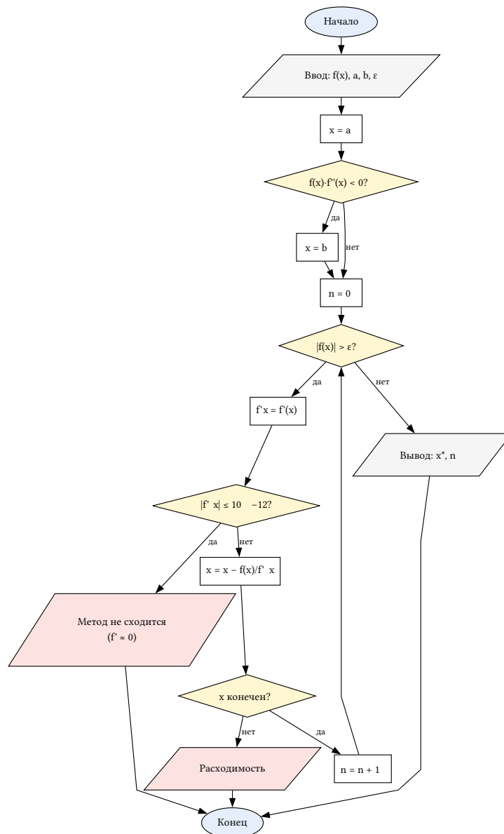
Рис. 2. Блок-схема метода Ньютона
