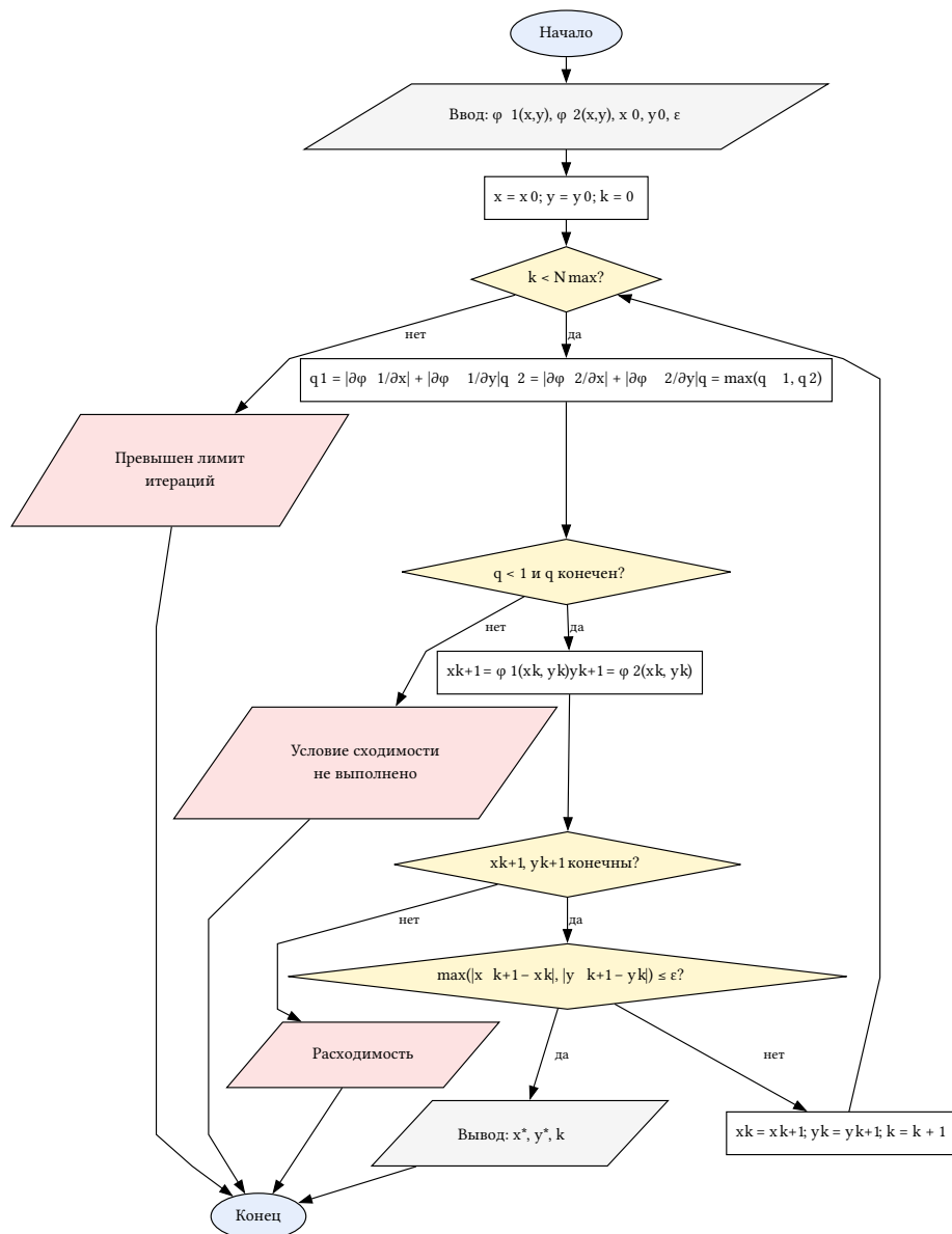
Рис. 4. Блок-схема метода простой итерации для системы
