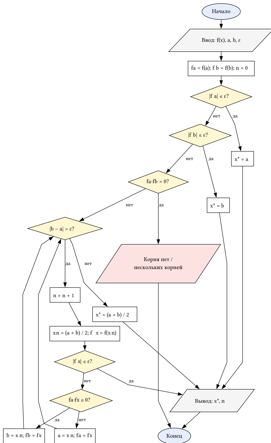
Рис. 1. Блок-схема метода половинного деления
