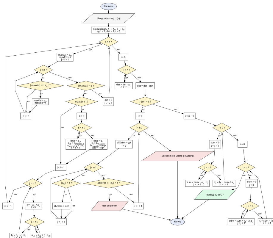
Рис. 1. Блок-схема метода Гаусса с выбором ведущего по столбцу
