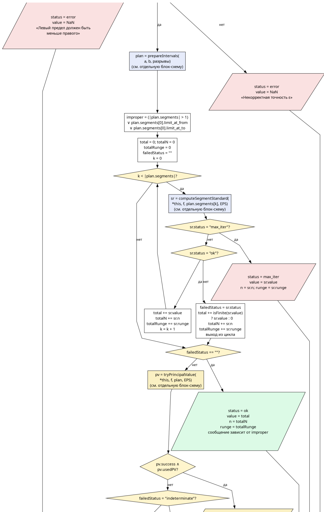
Рис. 7. Верхнеуровневая схема Integrator::integrate (подпрограммы — отдельные блок-схемы)
