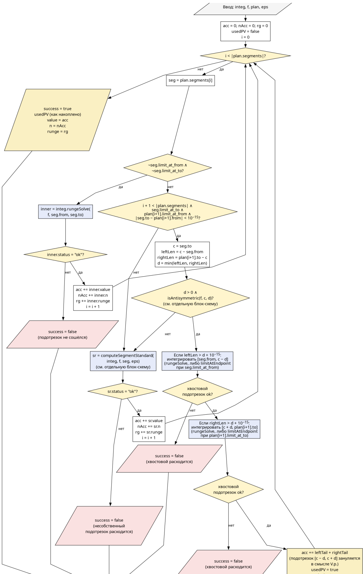
Рис. 11. tryPrincipalValue — fallback на главное значение Коши
