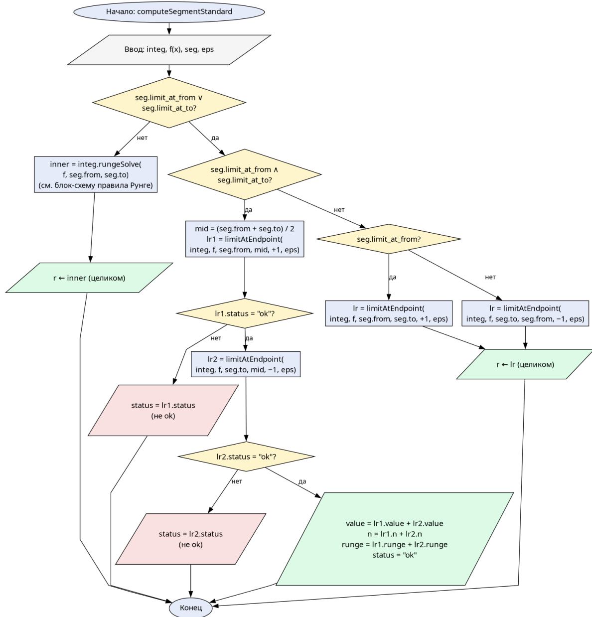
Рис. 9. computeSegmentStandard — выбор пути для одного сегмента
