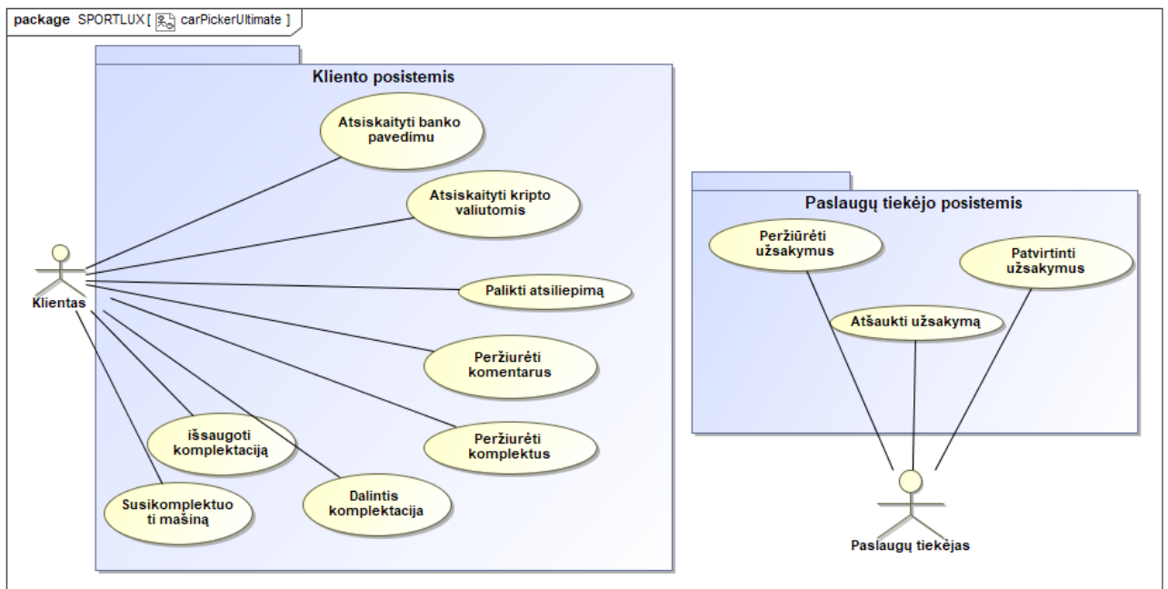
1 pav. „carPickerUltimate“ panaudojimo atvejų diagrama
