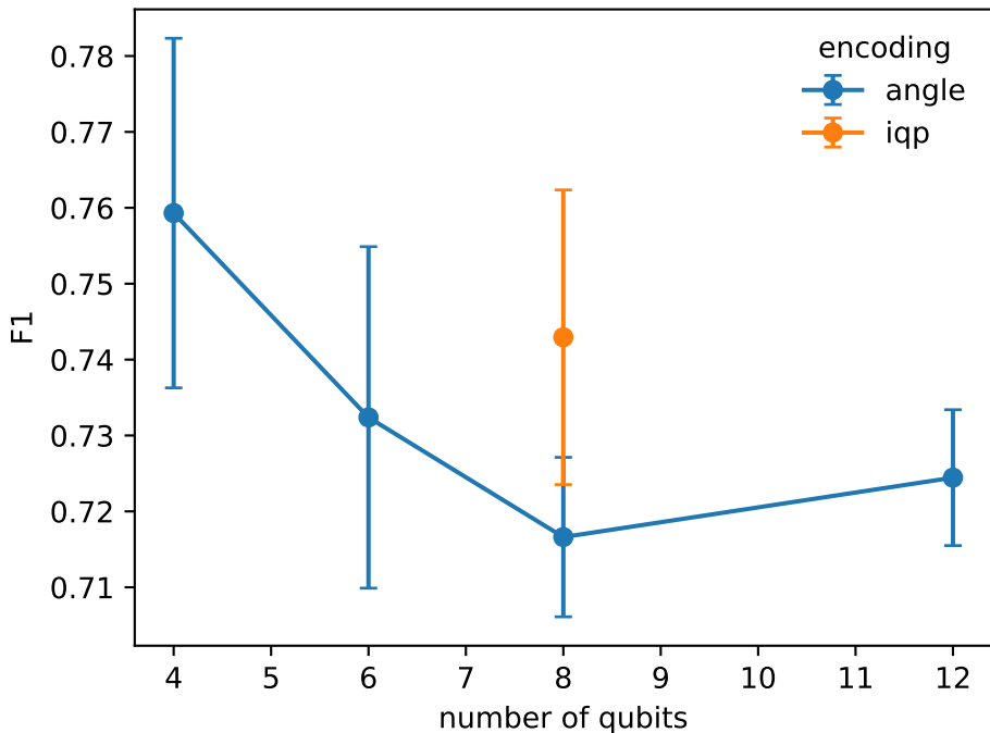
nskkdd: HybridQNN F1 vs qubits
