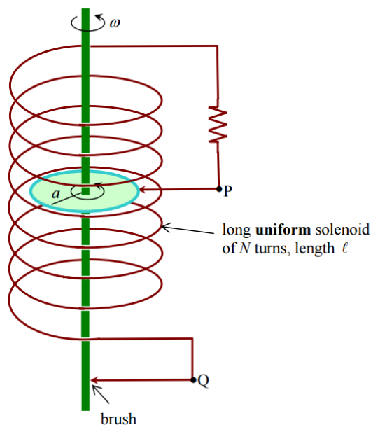
Figura 3.21: Auto dinamo
