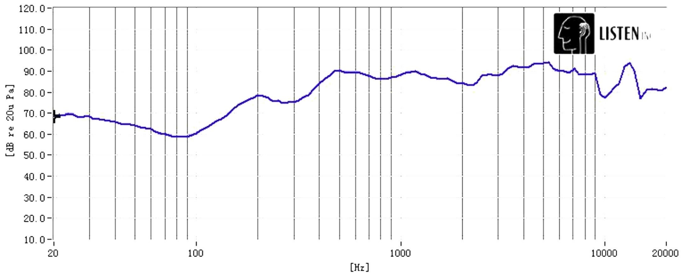
频响曲线
