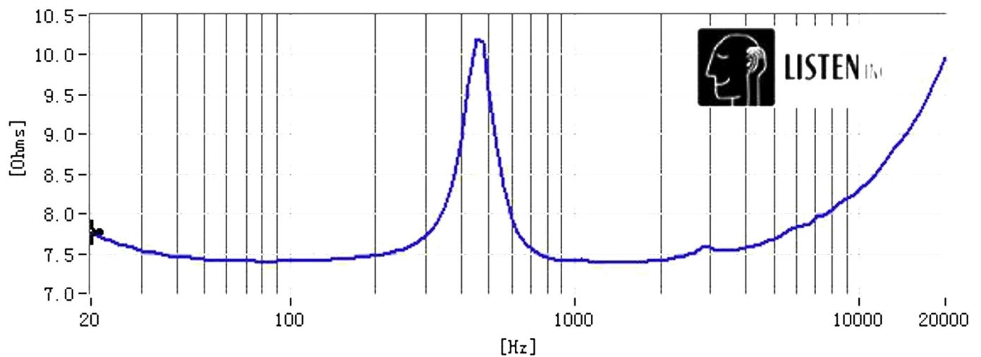
阻抗曲线
