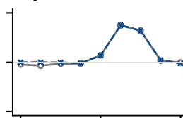
Layer 15 · ch 397
