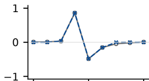
Layer 5 · ch 7
