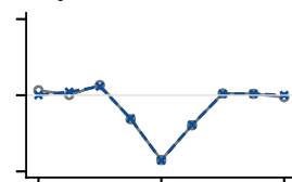
Layer 12 · ch 144
