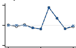
Layer 14 · ch 681
