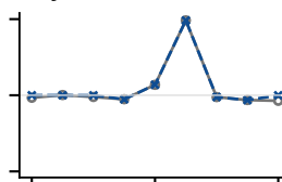
Layer 11 · ch 278
