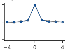
Layer 22 · ch 851
