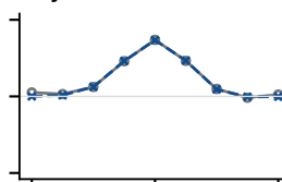
Layer 19 · ch 574
