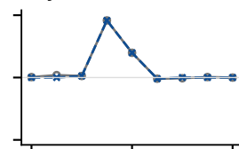
Layer 4 · ch 467
