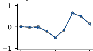
Layer 13 · ch 506
