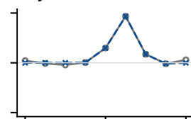
Layer 16 · ch 969
