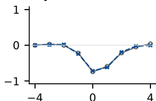
Layer 21 · ch 930
