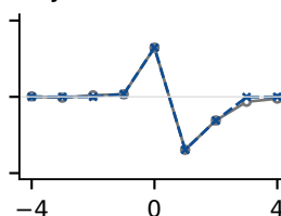
Layer 23 · ch 819
