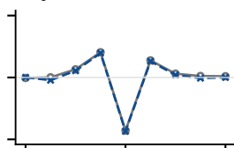
Layer 10 · ch 478
