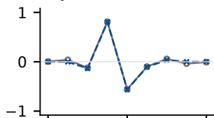
Layer 9 · ch 558
