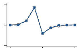
Layer 8 · ch 393
