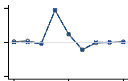
Layer 6 · ch 813
