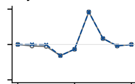
Layer 20 · ch 80
