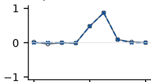
Layer 1 · ch 411
