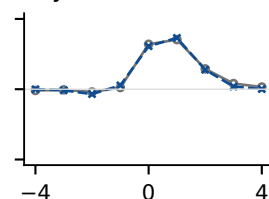
Layer 24 · ch 52
