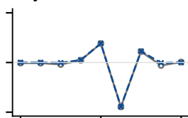
Layer 18 · ch 561
