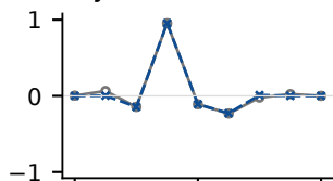
Layer 17 · ch 240
