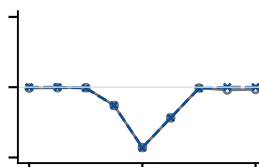
Layer 7 · ch 510
