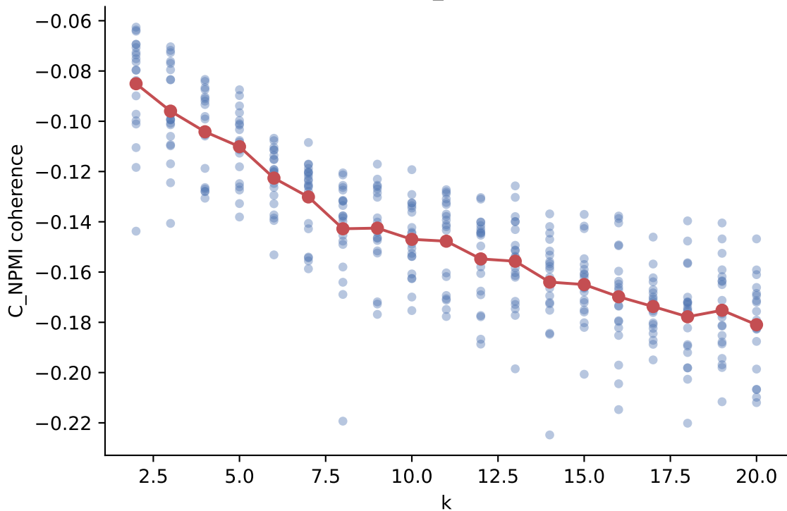
M2: metadata C_NPMI vs k (N=66)
