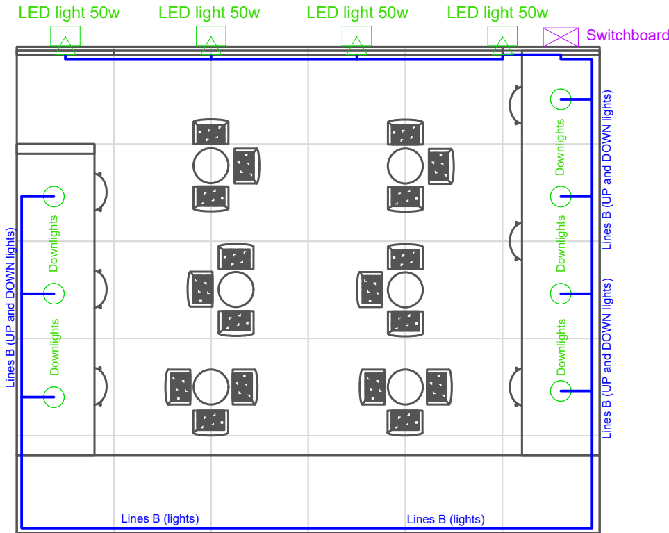
VISTA PLANTA (TECHO)
