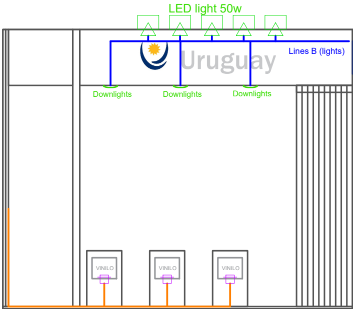
VISTA ALZADO LAT. IZQUIERDO
