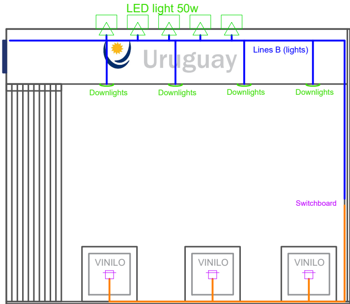
VISTA ALZADO LAT. DERECHO
