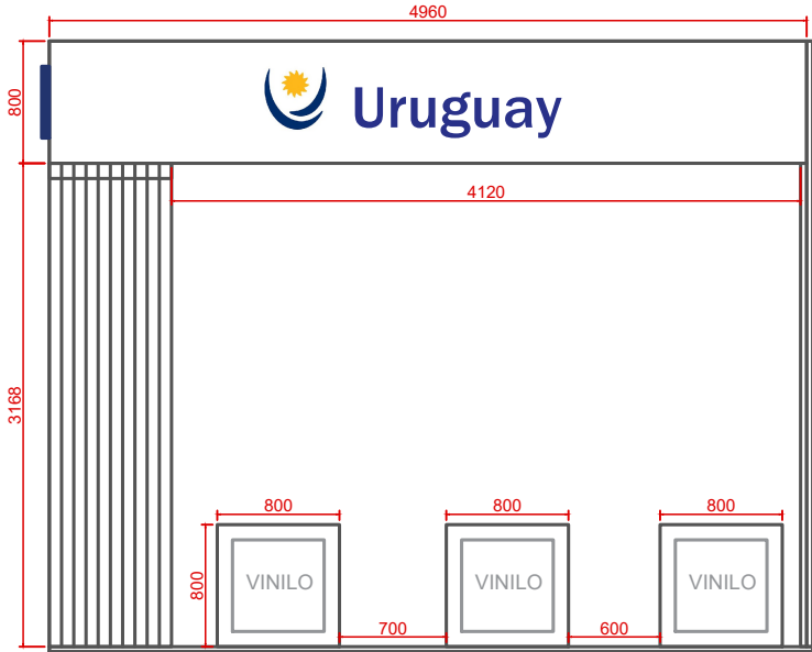
VISTA ALZADO LAT. DERECHO
