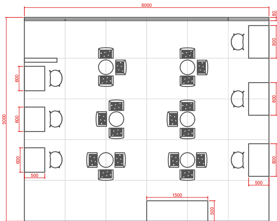
VISTA PLANTA (SUELO)
