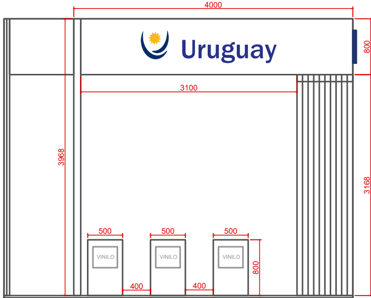
VISTA ALZADO LAT. IZQUIERDO
