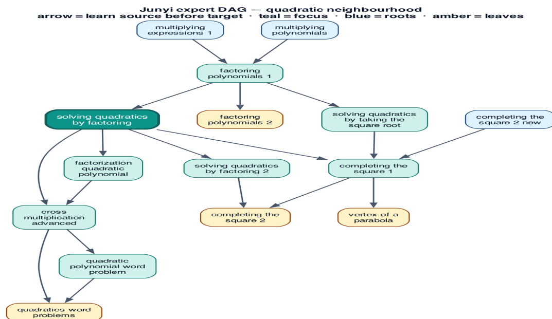
dag_quadratic.png
