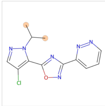
Molécula generada
