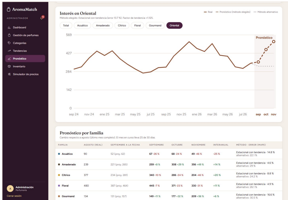
Figura 13. Pronóstico de Oriental: histórico de 24 meses, pronóstico del método elegido (línea discontinua) y método alternativo (punteada).
