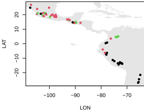
K=3
