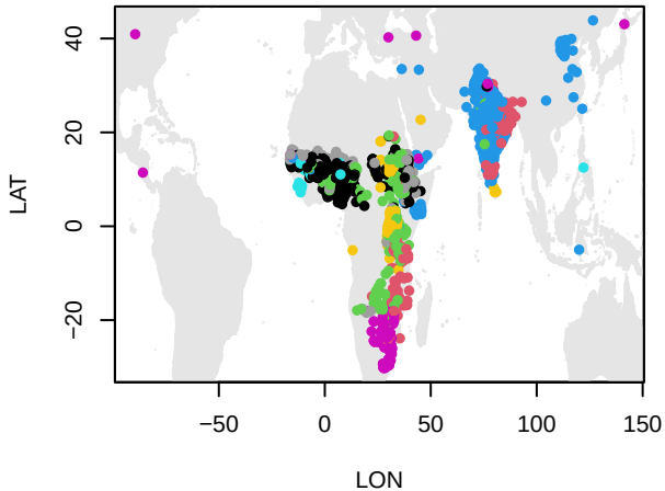
K=9
