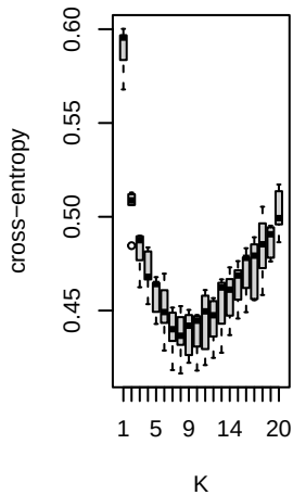
tomato_wr
