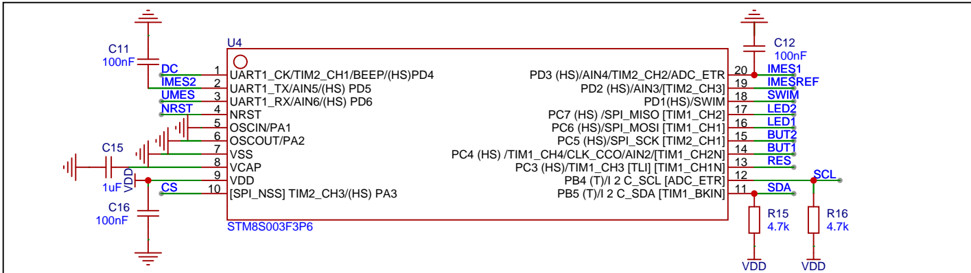
MCU 系统
