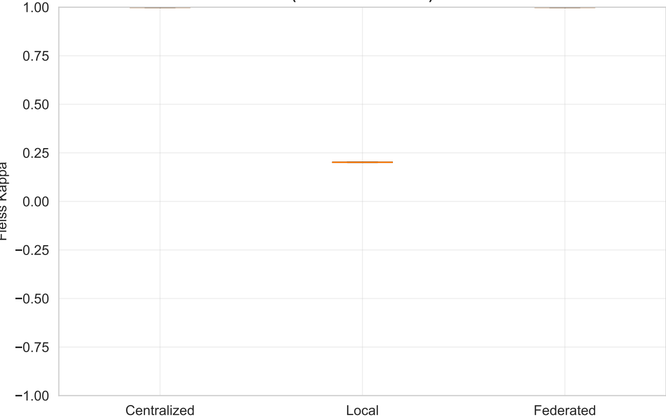
Fleiss Kappa: NerveDysesthesia (Global Thresholds)
