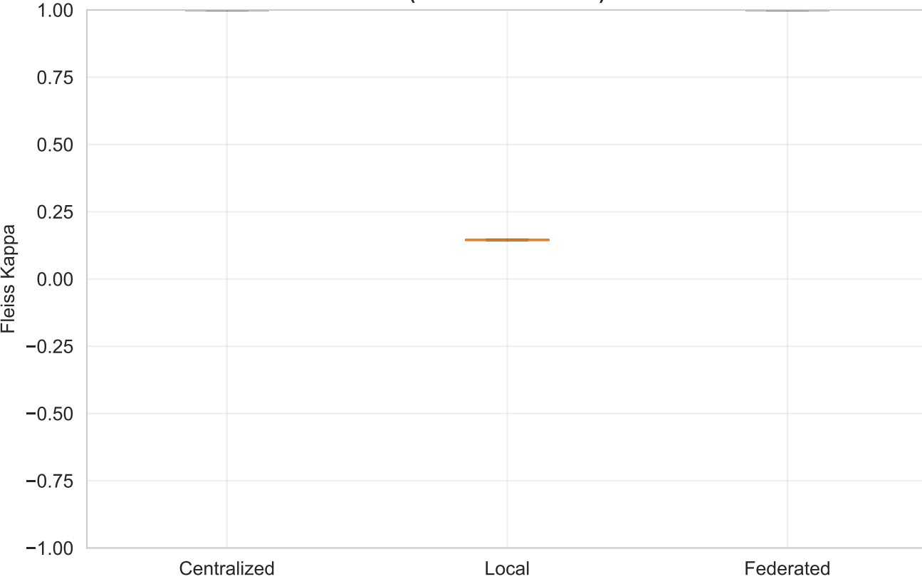
Fleiss Kappa: Bleeding (Global Thresholds)
