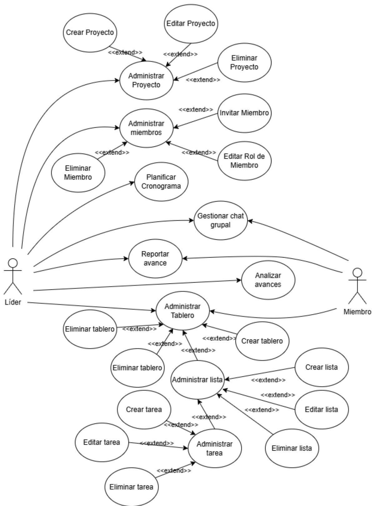
Figura 1. Diagrama de casos de uso de Plan-It.
