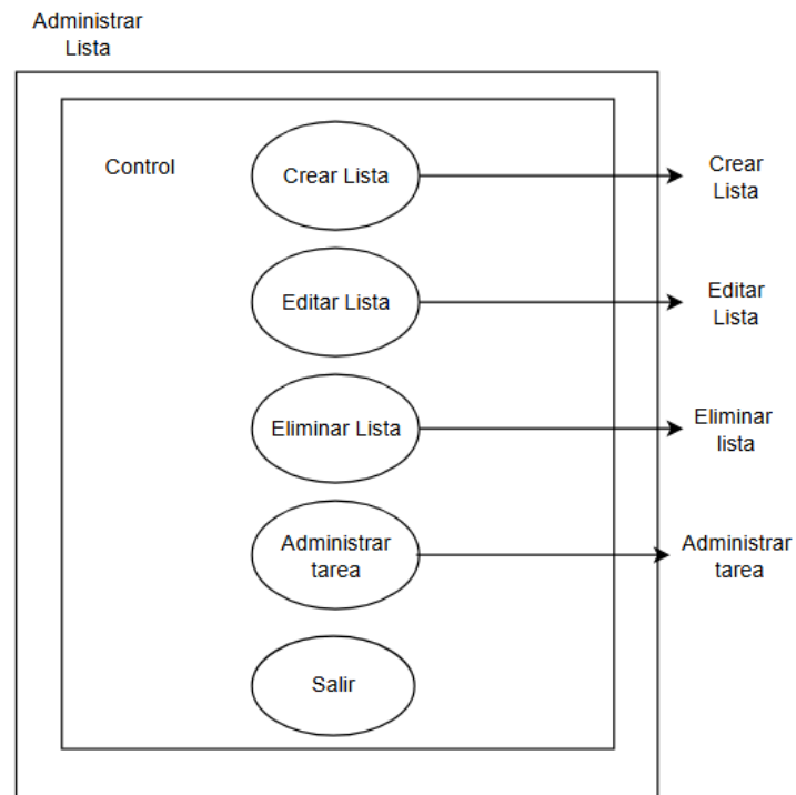
Figura 18: Especificación de componente “Administrar Lista”
