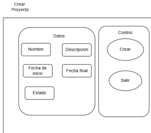
Figura 4: Especificación de componente "Crear Proyecto"
