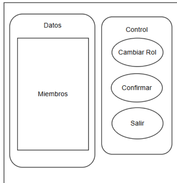
Figura 9: Especificación de componente "Editar rol de miembro"
