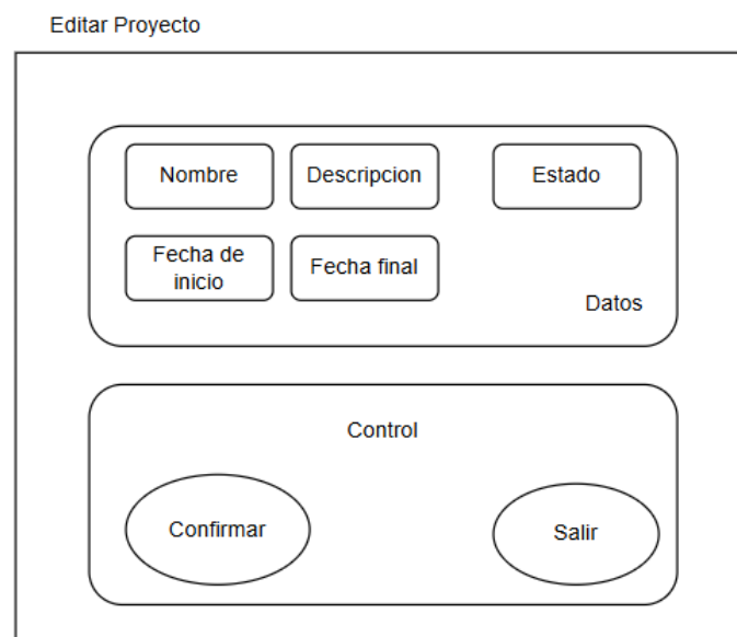
Figura 5: Especificación de componente "Editar Proyecto"
