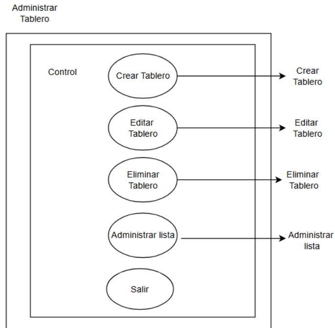
Figura 14: Especificación de componente “Administrar Tablero”
