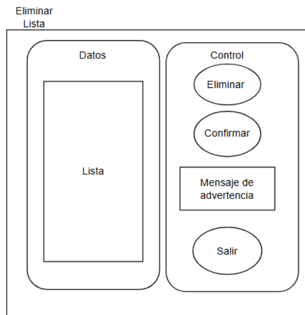
Figura 21: Especificación de componente "Eliminar Lista"
