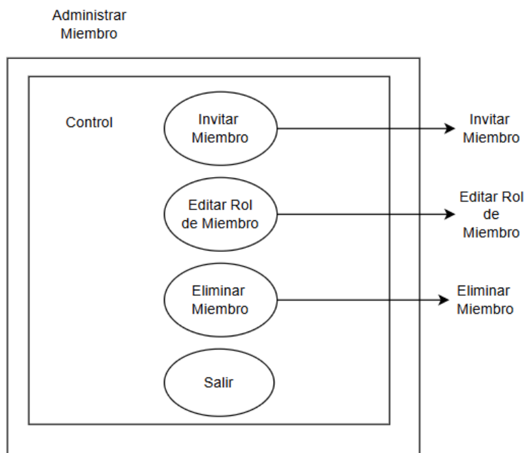
Figura 7: Especificación de componente “Administrar Miembro”
