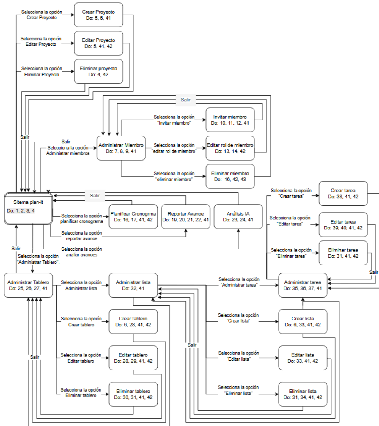
Figura 2: Diagrama de Diálogo de Plann-It
