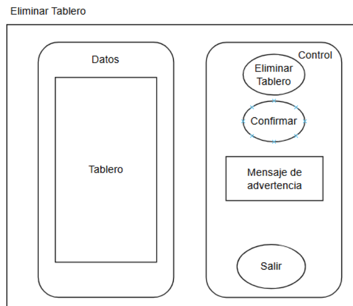
Figura 17: Especificación de componente “Eliminar Tablero”
