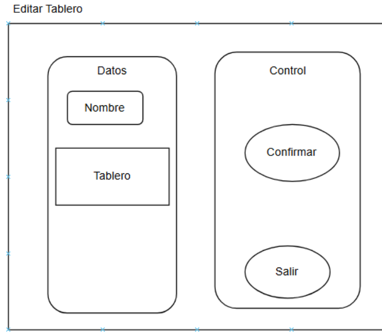
Figura 16: Especificación de componente “Editar”
