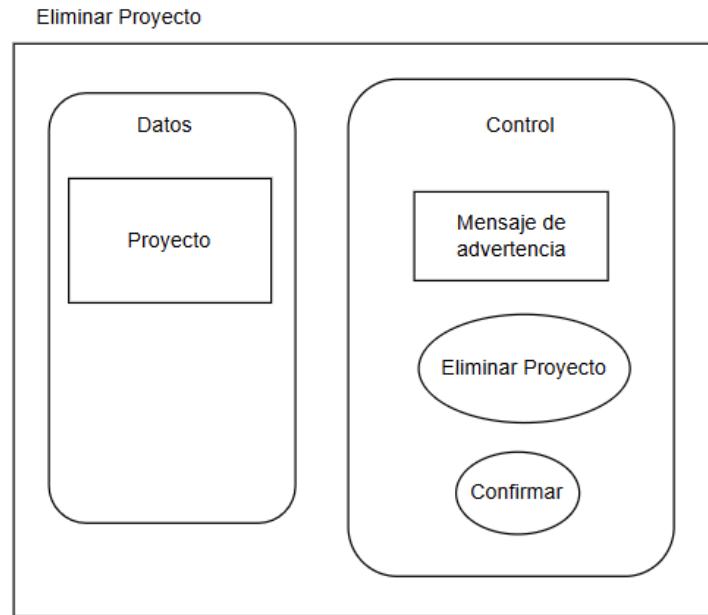
Figura 6: Especificación de componente “Eliminar Proyecto”
