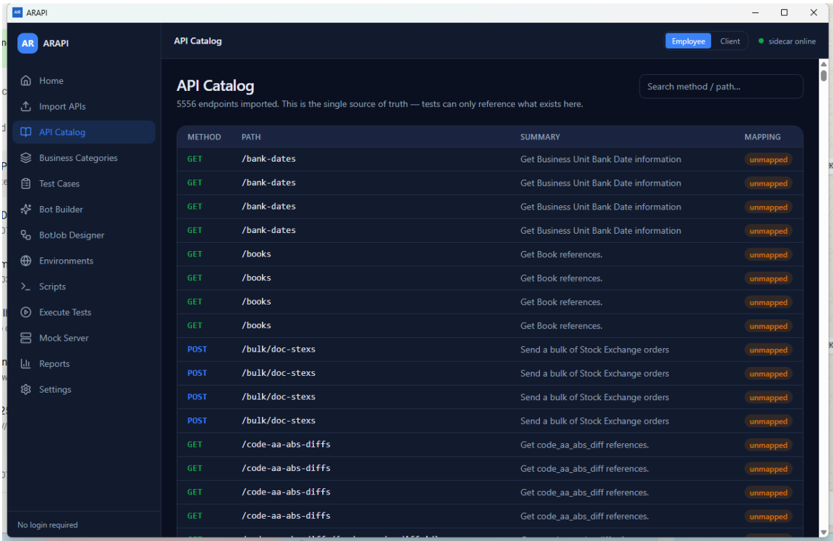
Figure 4. API Catalog
