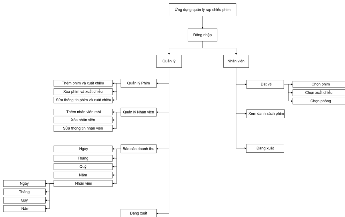
Hình 3.2.1: Sơ đồ thiết kế chức năng hệ thống
