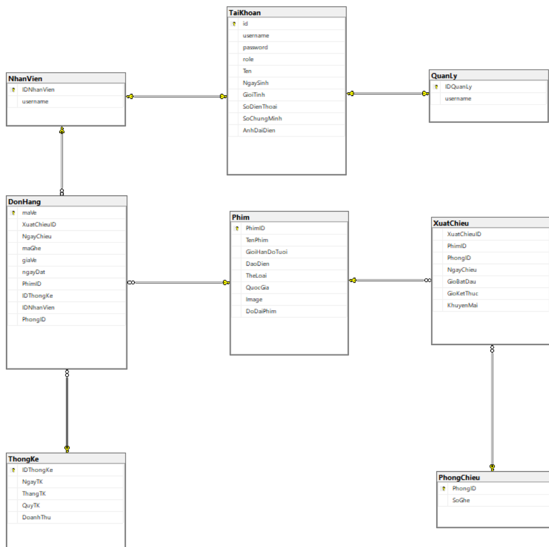
Hình 3.3.1: Sơ đồ dữ liệu quan hệ
