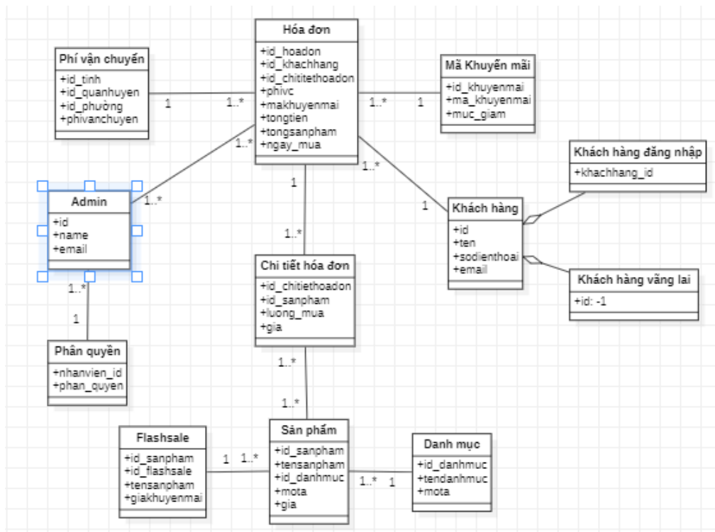
Hình 2: Class diagram
