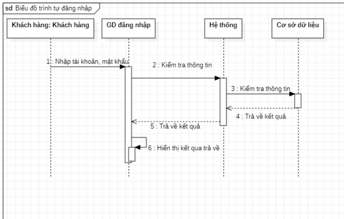
Hình 4: Sequence diagram
