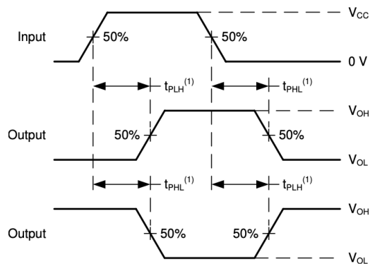
Abbildung 2: Definition der Verzögerungszeiten aus dem Datenblatt des IC [SNx4HC00]
