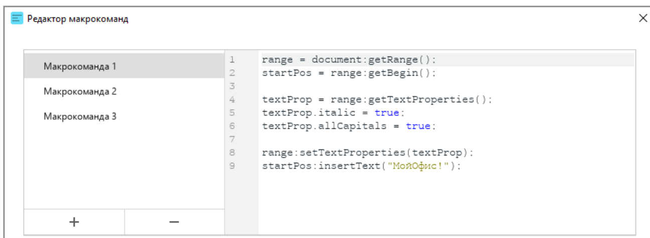
Рисунок 274 – Редактор макроккоманд
