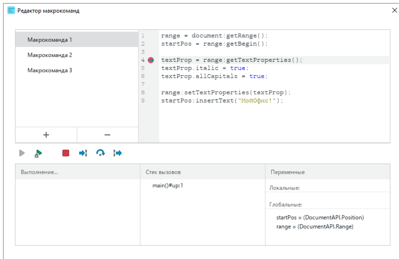
Рисунок 276 – Отладка макрокоманды
