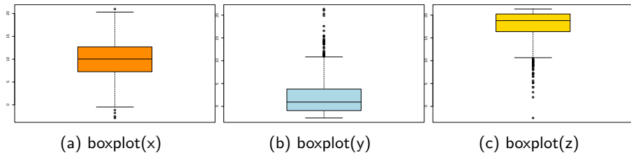
Figure 12: Distribuzioni a confronto
