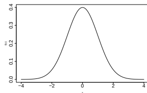
(a) Densità
