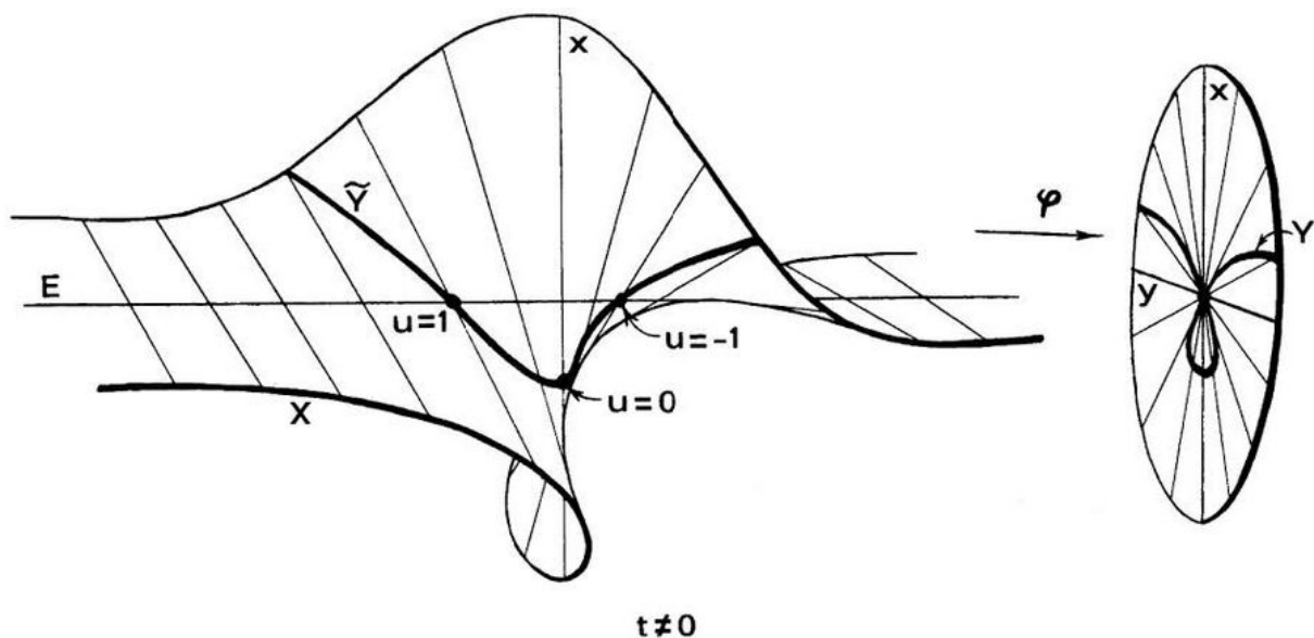
图 10.1.: 爆破的一个经典局部示意图. 态射 \varphi: \tilde{X} \rightarrow X 在中心 y 之外是同构, 而例外除子 E = \varphi^{-1}(y) 记录逼近方向; \tilde{Y} 表示 Y 的严格变换. 这张图只负责给直观; 不要把它当成度量模型或全局模型.
