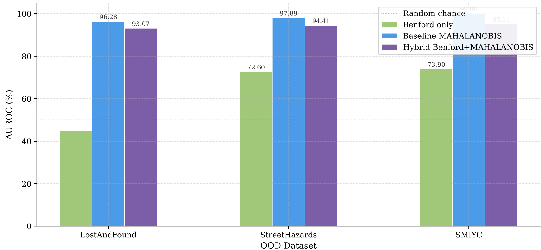
AUROC (%)
