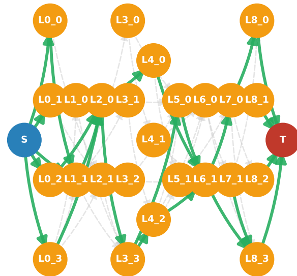
G' — Optimized 30 / 65 edges (46%) is_dspg=True
