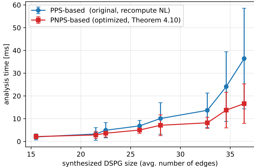
DSPG analysis time (same input DSPG)
