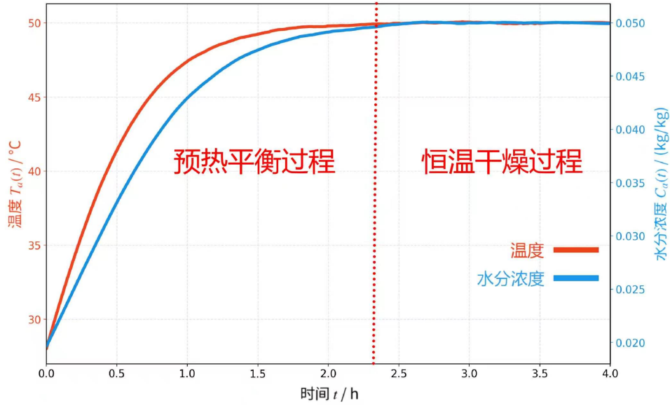
图 10 药材预热烘干过程示意图
