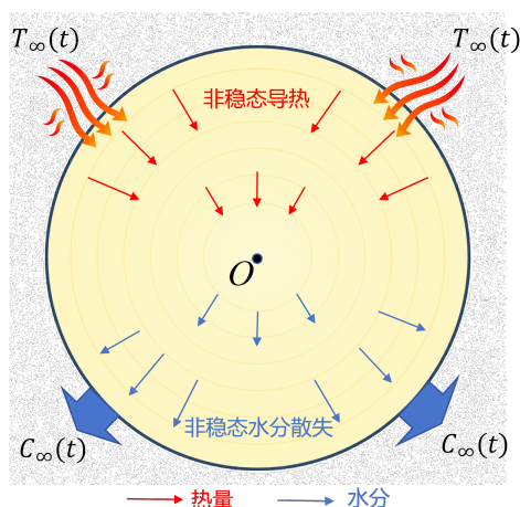
图 2 药材径向传热传质示意图
