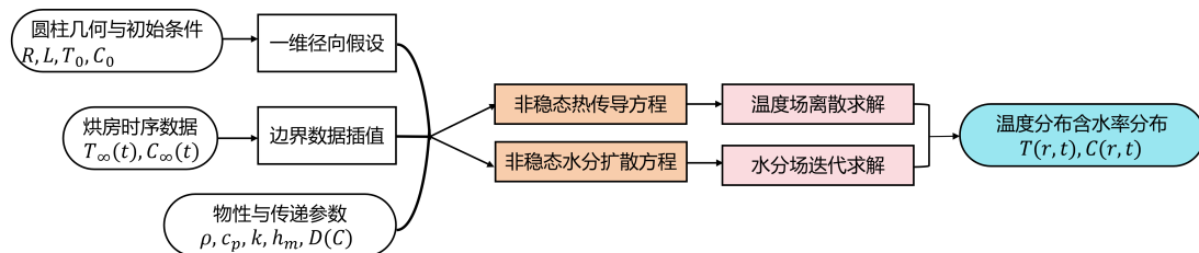
图3 问题一流程图
