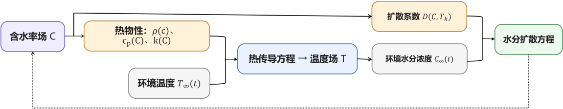
图 8 问题二热湿耦合计算流程图
