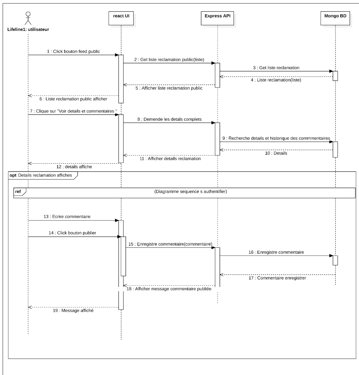
Figure 9 — DS-05 : Consultation des réclamations publiées et commentaires (BF5)
