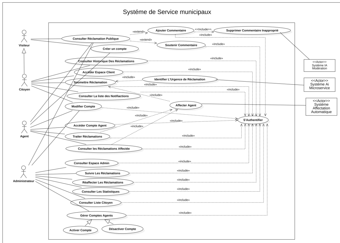
Figure 2 — Diagramme de Cas d'Utilisation Sprint 1
