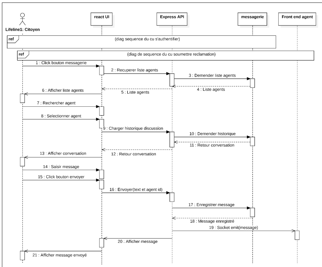
Figure 25 — DS-10 : Espace de messagerie (BF11)
