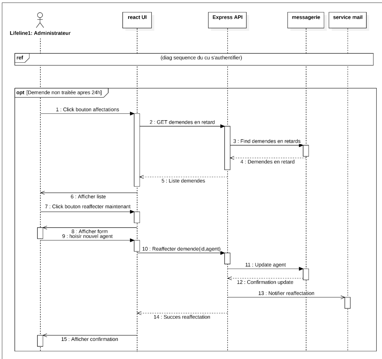
Figure 23 — DS-09 : Traitement des demandes des services (BF9)
