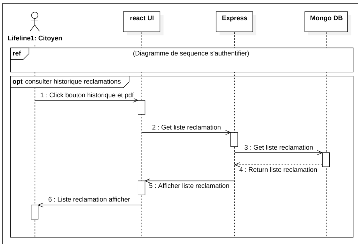
Figure 8 — DS-04 : Consultation De l'Histoire des réclamation (BF4) — Analyse texte par IA, masquage automatique si contenu inapproprié détecté.
