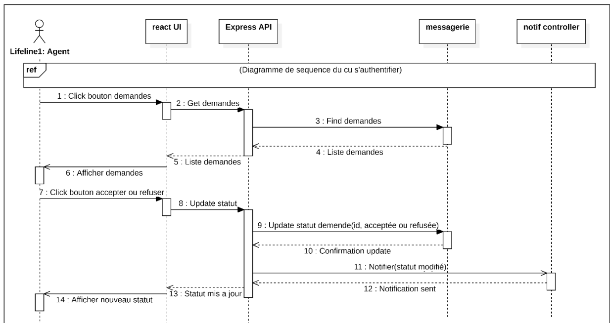
Figure 22 — DS-08 : Notifications par email (BF8) — Mise à jour statut + email notification citoyen.
