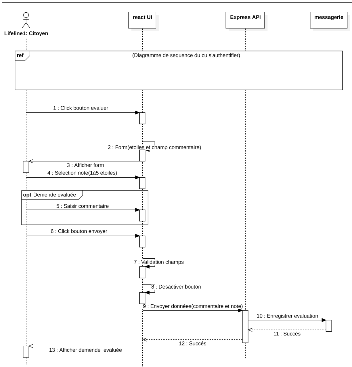
Figure 24 — DS-10 : Consultation des demandes et évaluation (BF10)
