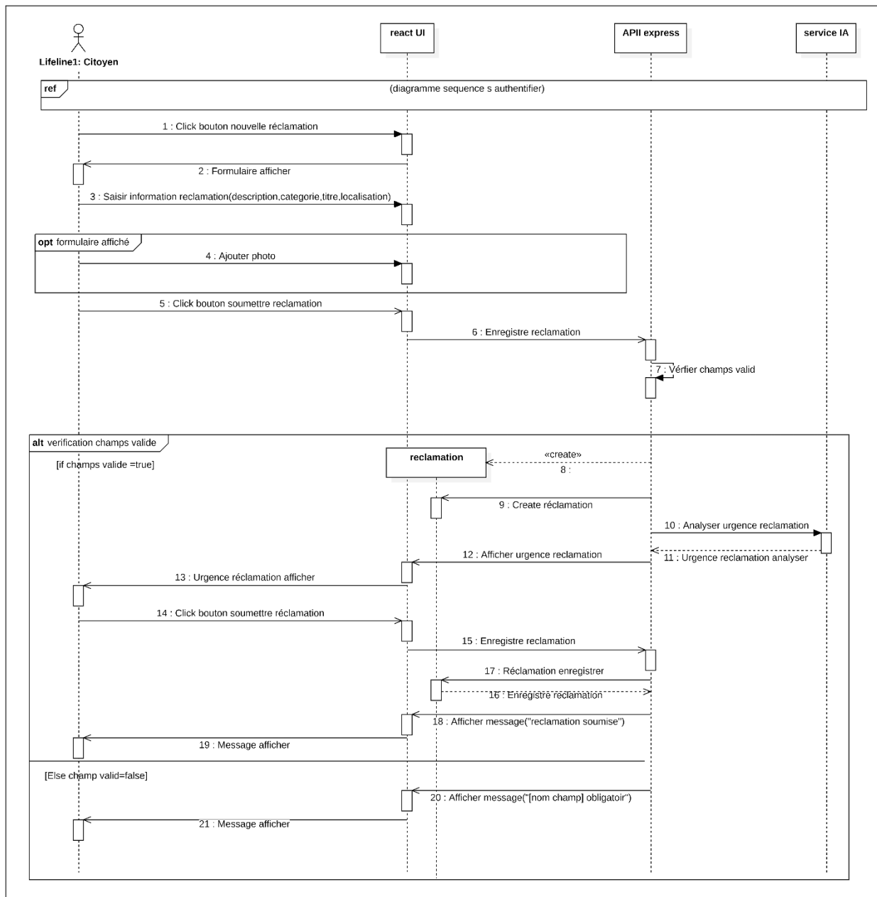
Figure 5 — DS-02 : Soumission Réclamation avec IA (BF2) — POST /predict au microservice Flask, intégration urgence, email Nodemailer.
