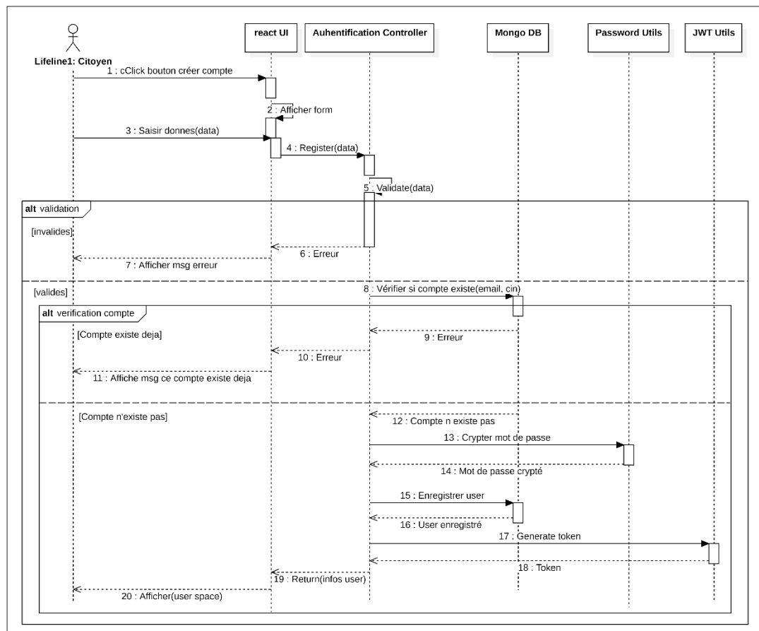
Figure 4 — DS-01 : Inscription et Connexion (BF1) — Hachage bcrypt, génération JWT, redirection par rôle.
