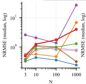
(a) Glycolysis/4-state
