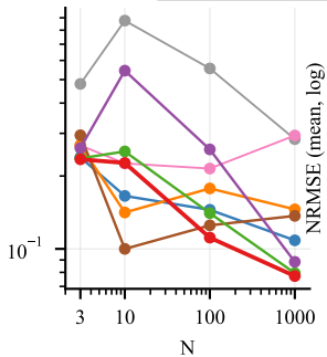
(a) Glycolysis/4-state
