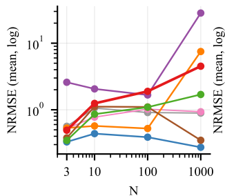
(d) Glycolysis/4-state
