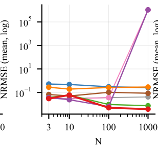
(h) Enzyme/4-state
